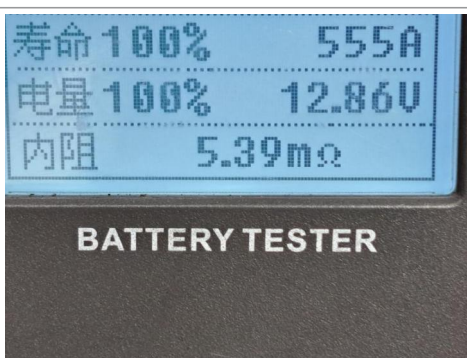
電瓶電壓
